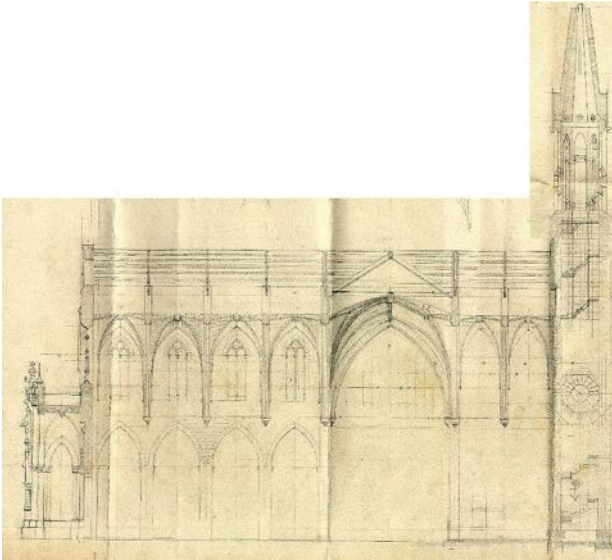
Secció longitudinal de l'església. Guillem Reynés, AGR
