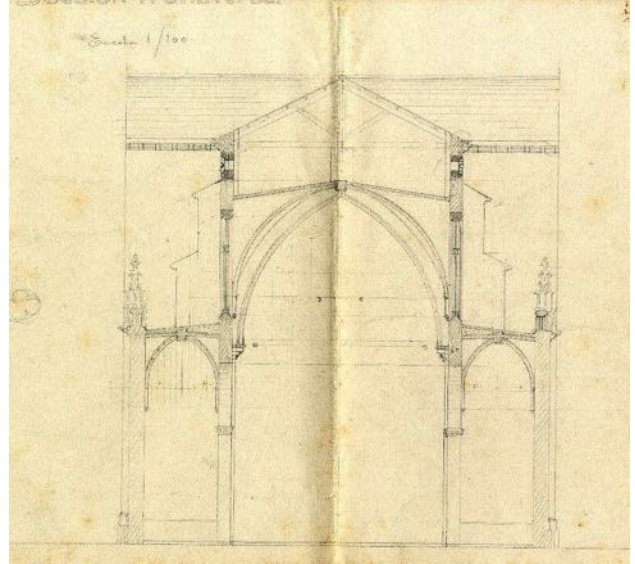
Secció transversal de la nau i les capelles de l'església. Guillem Reynés, AGR
